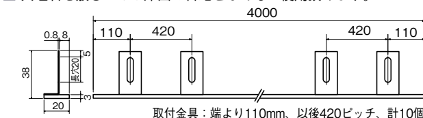
取付金具: 端より110mm、以後420ピッチ、計10個
